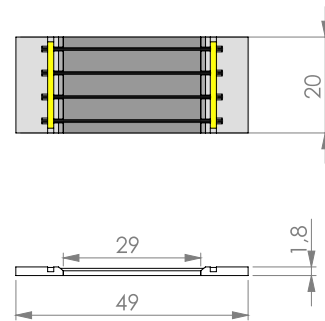
M2920E10 – Actuator Module only
